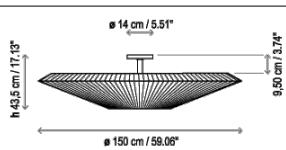
Bover SIAM подвесной
