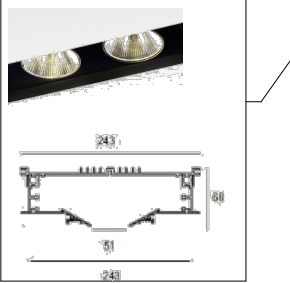
Delta Light Splitline 51 встраиваемая профильная система
